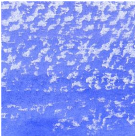
1、梅雨明けの巻積雲 紙の粗目を生かして ソフトパステルで描きます
